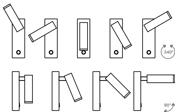
Lector orientable con doble movimiento de hasta 340° y 90° Adjustable reader with double movement up to 340° and 90° Lecteur réglable avec double mouvement jusqu'à 340° et 90°
