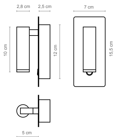
Manhattan a empotrado Manhattan a recessed Manhattan a encastrable
