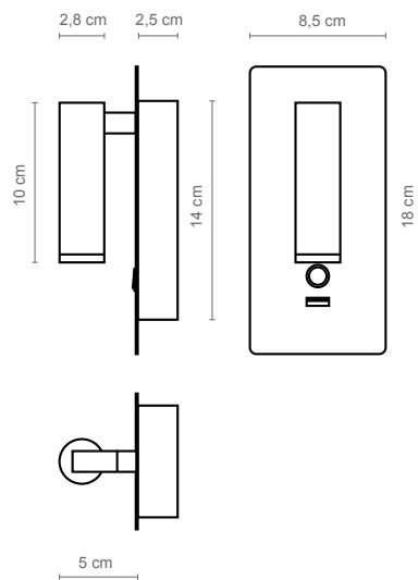
Manhattan a empotrado con USB Manhattan a recessed with USB Manhattan a encastrable avec USB
