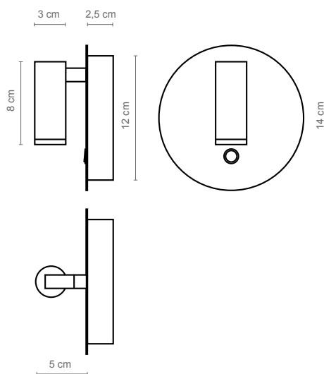
Manhattan a circular de superficie con lector mini Manhattan a circular surface-mounted with mini-reader Manhattan a circulaire en surface avec mini-lecteur
