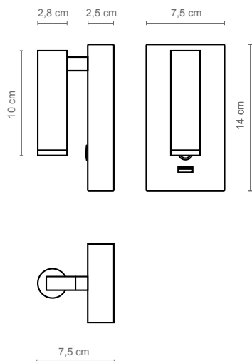
Manhattan a de superficie con USB Manhattan a surface-mounted with USB Manhattan a en surface avec USB
