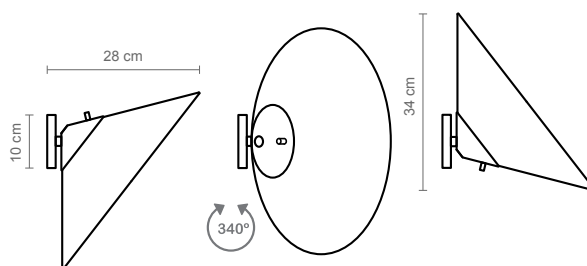
Cim a con movimiento rotatorio de hasta 340°
