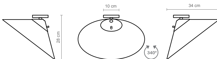
Cim a con movimiento rotatorio de hasta 340°
