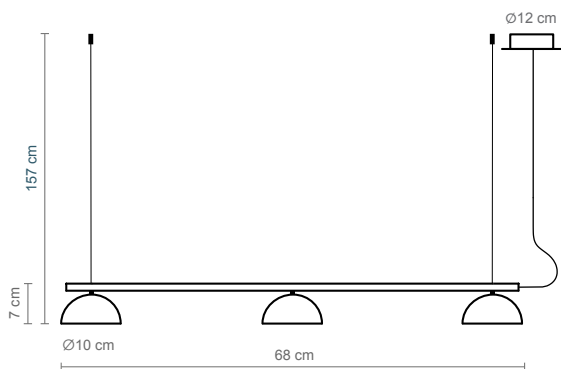
Absidiola c lineal 3 MINI
