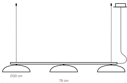
Absidiola c lineal 3 PLATO
