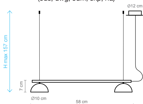
Absidiola c lineal 2 MINI
